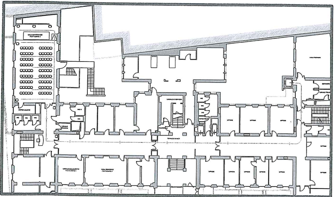
PIANO PRIMO
