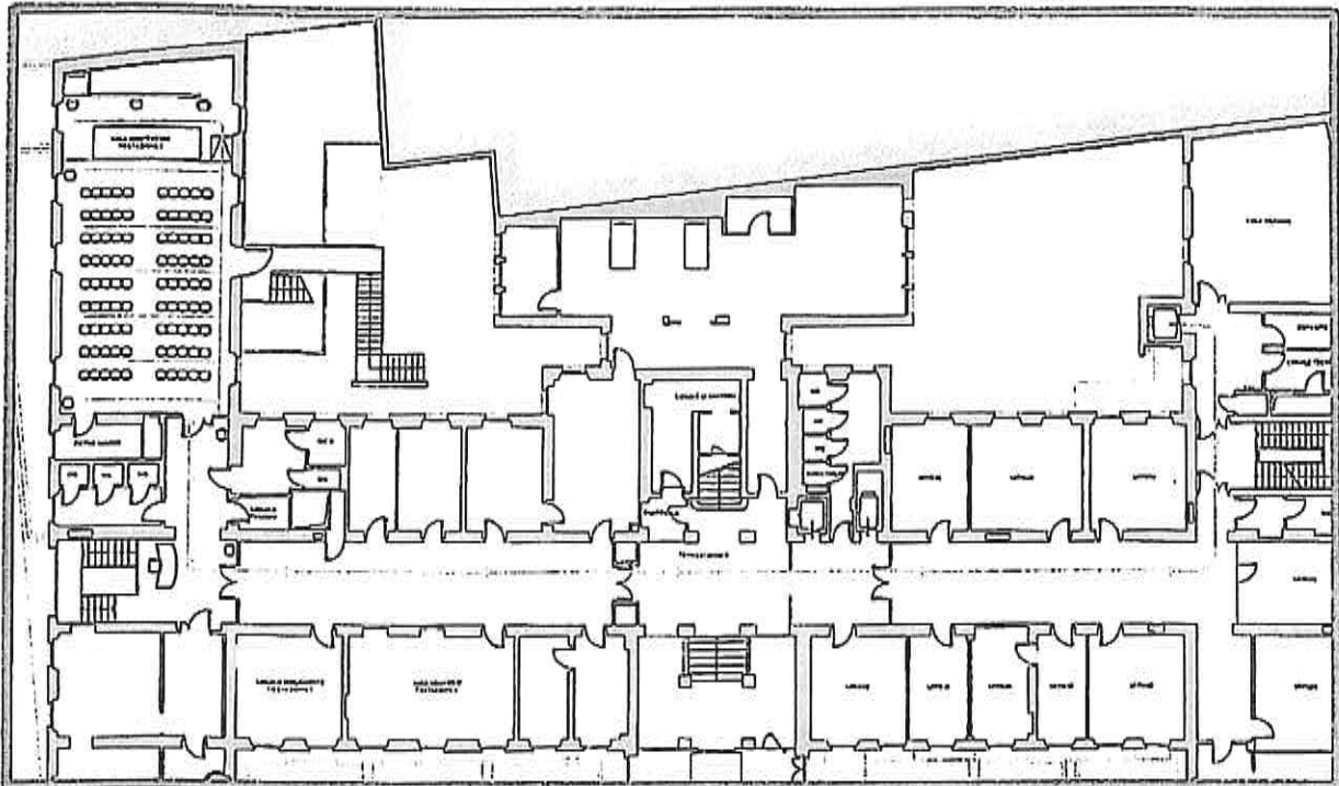
PIANO PRIMO
